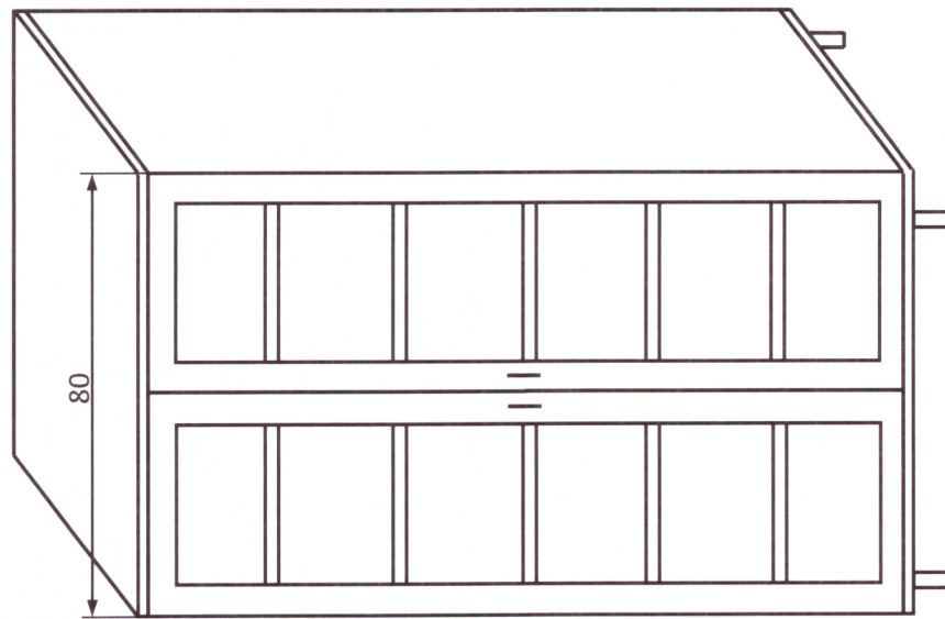
rzut główny
